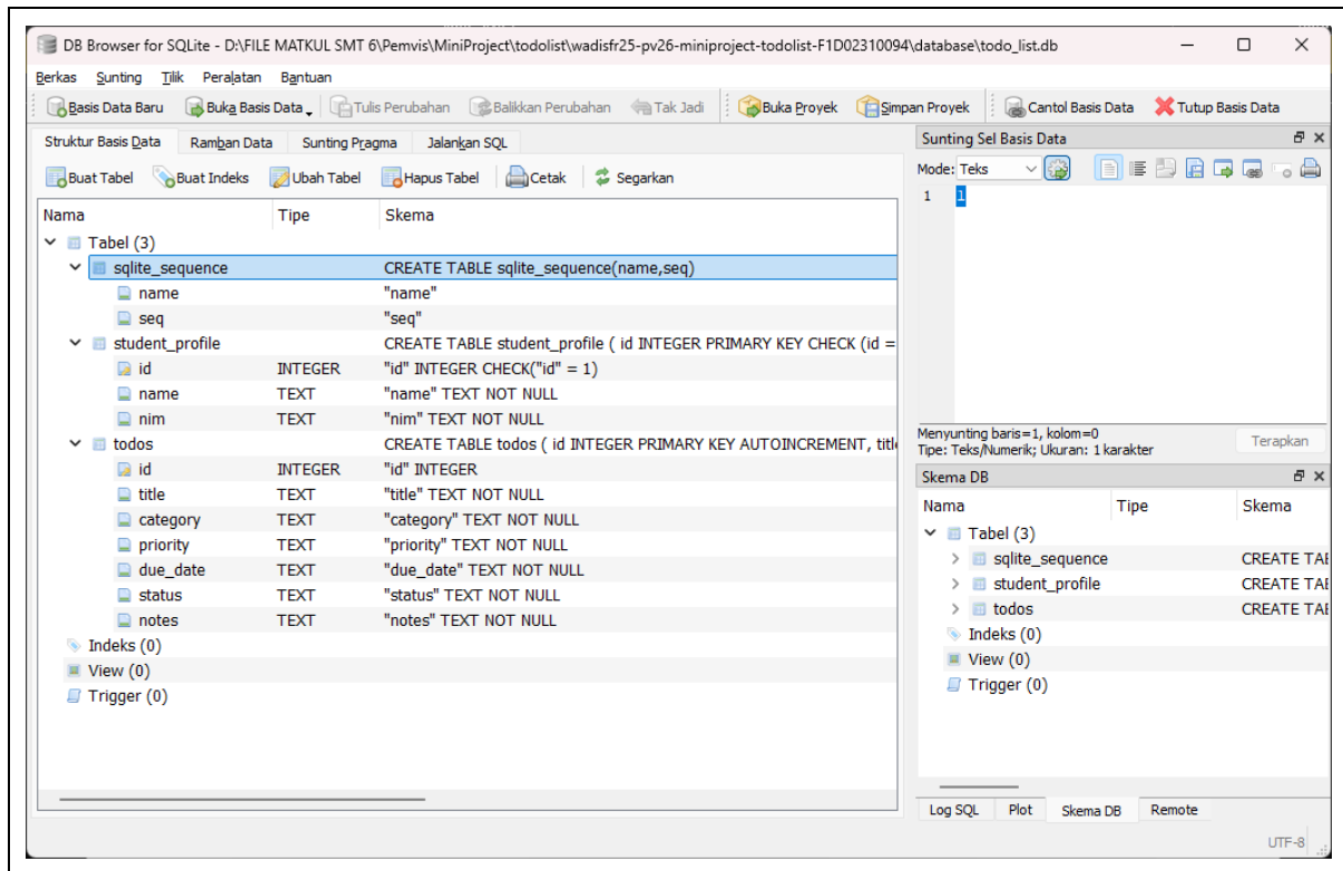
Gambar 3.1 Databsae Struktur
