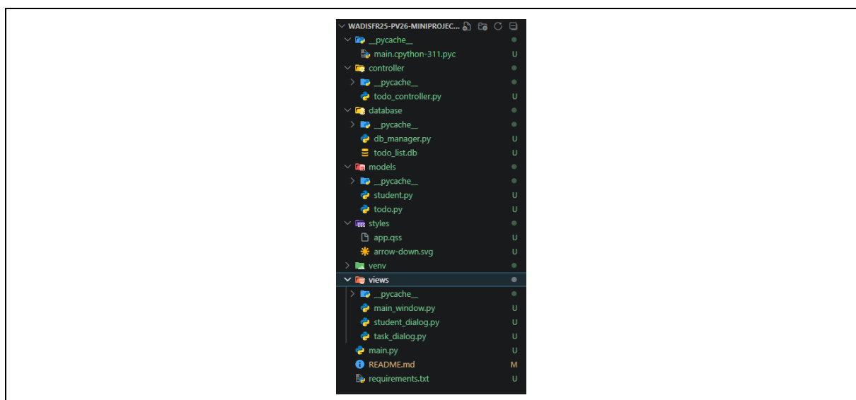
Gambar 2.1 Struktur Project
